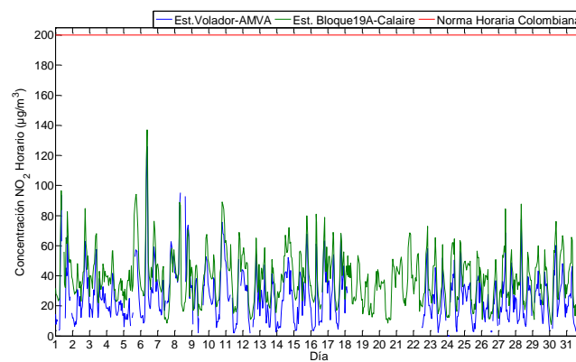
Figura 2. Concentración horaria de NO 2 – agosto de 2018.
