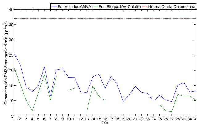
Figura 1. Concentración promedio diaria de PM2.5 – agosto de 2018.
