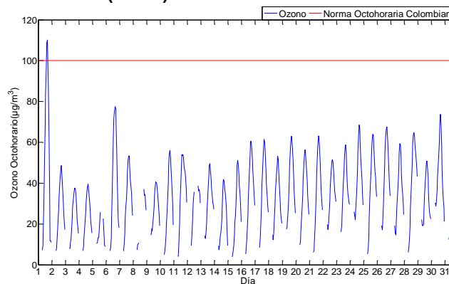
Figura 5. Concentración Octohoraria de O 3 , estación Universidad Nacional, El Volador – agosto de 2018.
