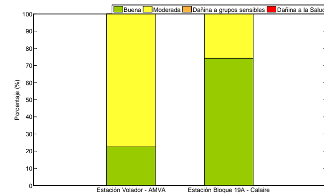
Figura 6. Índice de calidad de aire (ICA). Estaciones Universidad Nacional de Colombia – sede Medellín, agosto 2018.
