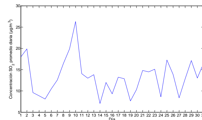
Figura 3. Concentración promedio diaria de SO 2 , estación MED-UNNP – agosto de 2018.
